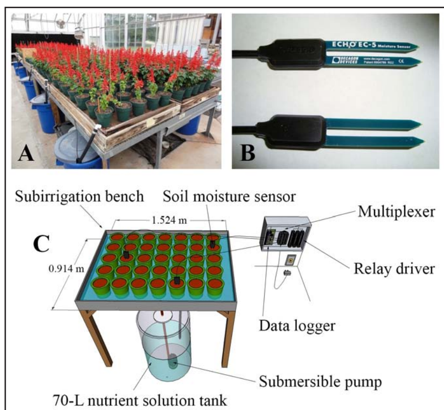
Figure 1. View of (A) subirrigation benches with Salvia splendens 'Vista Red' plants and 70 L-tanks (with submersible pumps inside), (B) EC-5 capacitance soil moisture sensor and (C) completely automated irrigation control system using capacitance-type sensors connected to a multiplexer, data logger and relay drivers [vista geral (A) das mesas de subirrigação com plantas de Salvia splendens 'Vista Red' e dos reservatórios de 70 L com as bombas submersas de irrigação no seu interior, (B) de um sensor capacitivo de umidade EC-5 e (C) do sistema de controle automatizado de irrigação utilizando sensores capacitivos de umidade conectados a um multiplexador, sistema automatizado de aquisição de dados e controlador de saídas]. Athens, University of Georgia, 2011.
